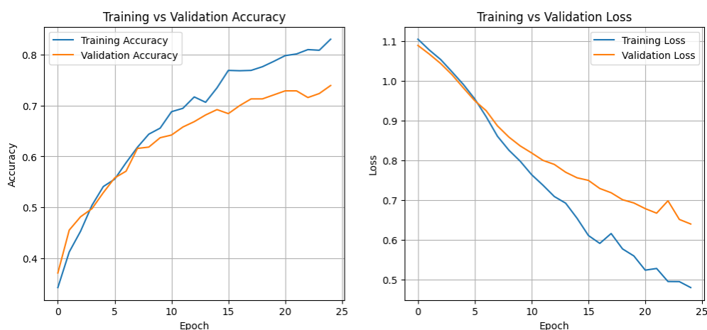
Gambar 4.14 Grafik Akurasi dan Loss Model LSTM
